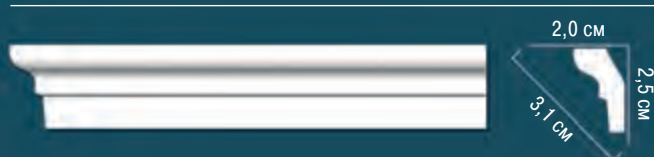
AB241, AB241F (гибкий)
